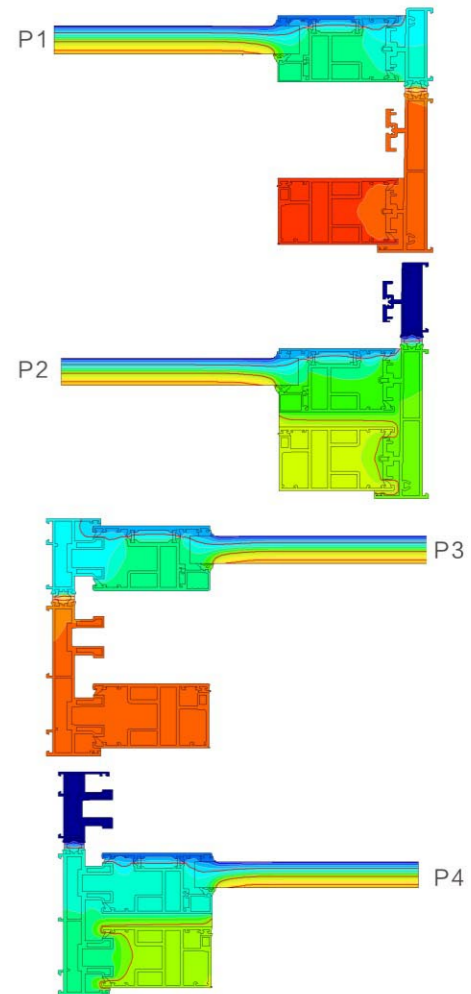
204三轨提升推拉门(带金刚网)热工图
